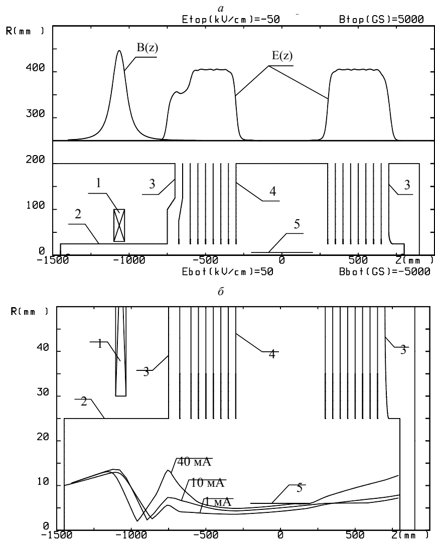
Рис. 4. Согласованный ввод 25 кэВ пучка H^- в ускоритель-тандем по «жесткой» схеме фокусировки: геометрия ионно-оптического тракта, расчетные осевые распределения полей (а) и огибающие ионных пучков с током 1 мА, 10 мА и 40 мА (б). Цифрами обозначены: 1 – катушка с током, 2 – трубка дрейфа, 3 – вакуумный бак, 4 – высоковольтный электрод, 5 – перезарядная трубка.
