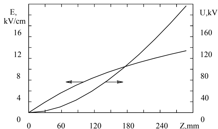
Рис. 5. Аналитическое распределение потенциала U и поля E , которое обеспечивает ускорение пучка отрицательных ионов водорода с начальной энергией 25 кэВ и током 10 мА при постоянном диаметре 10 мм.
