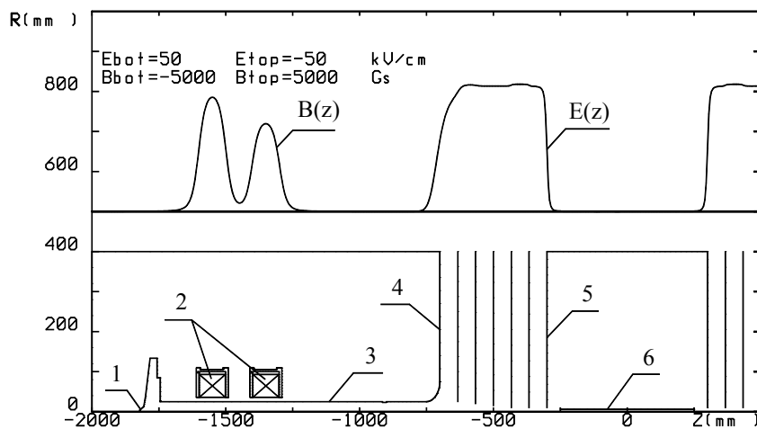
Рис. 12. Геометрия ионно-оптического тракта ускорителя-тандема и расчетное осевое распределение полей для схемы «жесткой» фокусировки пучка H^- с током 10 мА и начальной энергией 25 кэВ. Цифрами обозначены: 1 – ионный источник, 2 – магнитные линзы, 3 – трубка дрейфа, 4 – вакуумный бак, 5 – высоковольтный электрод, 6 – перезарядная трубка.
