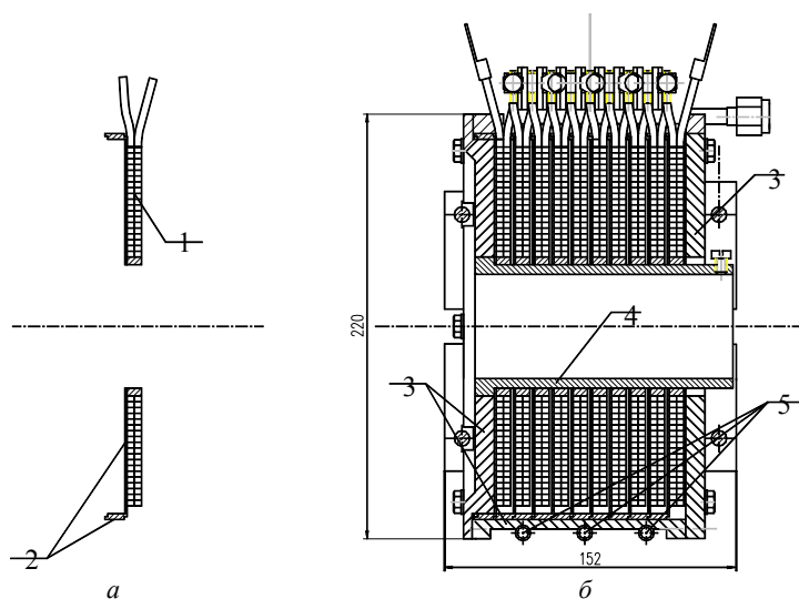
Рис. 8. Чертеж магнитной линзы: базовый модуль обмотки (а) и магнитная линза в сборе (б). Цифрами обозначены: 1 – шинка с током, 2 – алюминиевый диск, 3 – магнитный экран, 4 – каркас линзы (нержавеющая сталь), 5 – трубки системы охлаждения.
