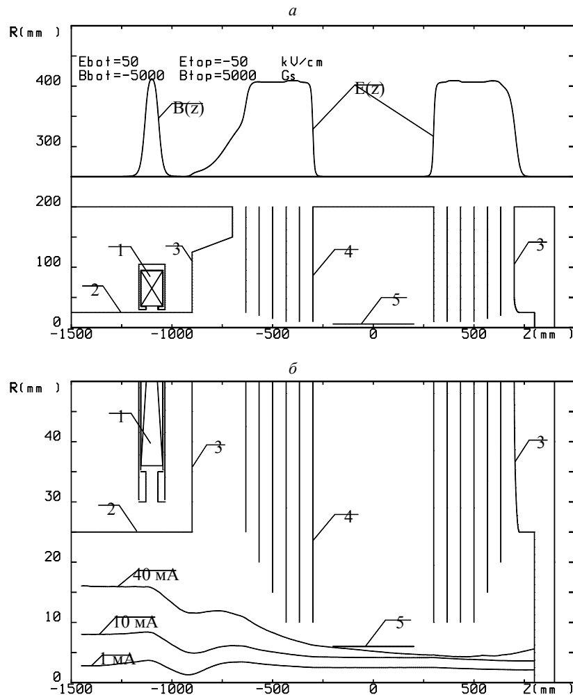
Рис. 7. Согласованный ввод 25 кэВ пучка H^- в ускоритель-тандем с использованием упрощенной схемы «мягкой» фокусировки: геометрия ионно-оптического тракта, расчетное осевое распределение полей (а) и огибающие ионных пучков с током 1 мА, 10 мА и 40 мА, охватывающие 95 % тока (б). Цифрами обозначены: 1 – магнитная линза, 2 – трубка дрейфа, 3 – вакуумный бак, 4 – высоковольтный электрод, 5 – перезарядная трубка.
