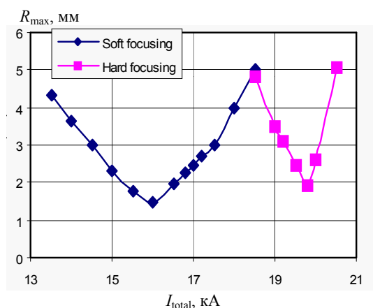
Рис. 14. Расчетная зависимость максимального радиуса огибающей 95% тока пучка H^+ в перезарядной трубке от полного тока во второй магнитной линзе для схем «мягкой» и «жесткой» фокусировки пучка
