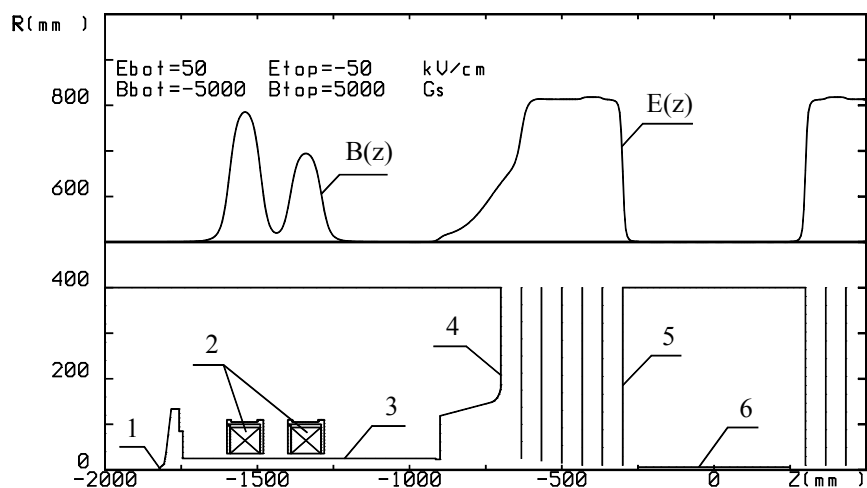
Рис. 10. Геометрия ионно-оптического тракта ускорителя-тандема и расчетное осевое распределение полей для схемы «мягкой» фокусировки пучка H^+ с током 10 мА и начальной энергией 25 кэВ. Цифрами обозначены: 1 – ионный источник, 2 – магнитные линзы, 3 – трубка дрейфа, 4 – вакуумный бак, 5 – высоковольтный электрод, 6 – перезарядная трубка.
