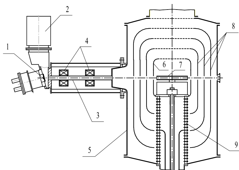
Рис.1. Схема 2,5 МэВ ускорителя-тандема: 1 – источник отрицательных ионов, 2 – вакуумный насос, 3 – трубка дрейфа, 4 – магнитные линзы, 5 – вакуумный бак, 6 – высоковольтный электрод, 7 – перезарядная трубка, 8 – промежуточные электроды, 9 – высоковольтный изолятор.
