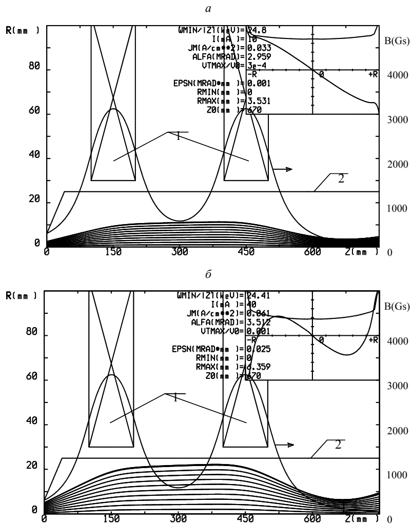
Рис.3. Транспортировка 25 кэВ пучка H + с током 10 мА (а) и 40 мА (б) с помощью двух магнитных линз: расчетные характерные траектории частиц и осевое распределение магнитного поля В. Цифрами обозначены: 1 – катушки с током, 2 – контур трубки дрейфа. На вставке в верхнем правом углу приведены радиальное распределение плотности тока и фазовый портрет пучка в фокусе второй линзы.
