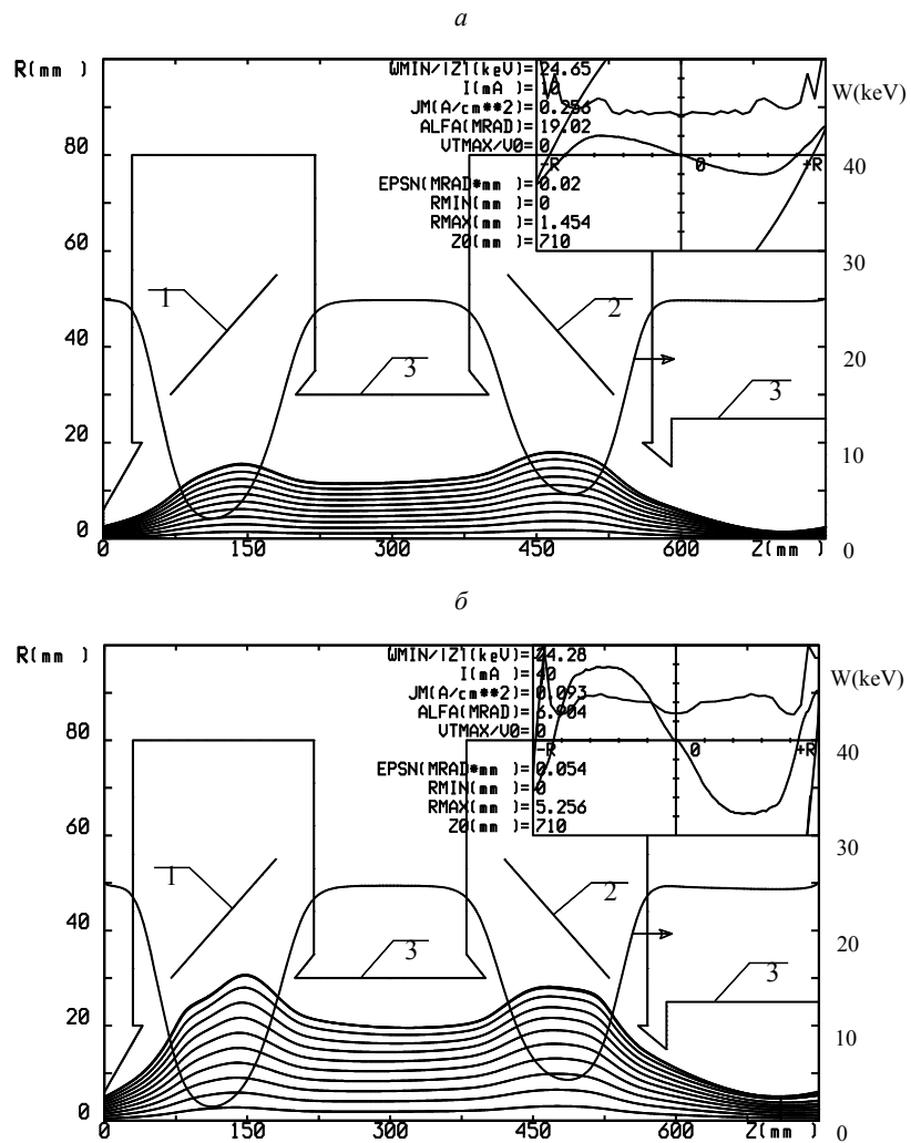
Рис.2. Транспортировка 25 кэВ пучка H^+ с током 10 мА (а) и 40 мА (б) с помощью двух электростатических линз: расчетные характерные траектории частиц и осевое распределение энергии ионов W . Цифрами обозначены: 1 – первый тормозящий электрод, 2 – второй тормозящий электрод, 3 – контур трубки дрейфа. На вставке в верхнем правом углу приведены радиальное распределение плотности тока и фазовый портрет пучка в фокусе второй линзы.
