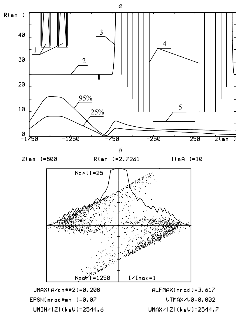
Рис. 13. Результаты расчета ионно-оптического тракта ускорителя-тандема для схемы «жесткой» фокусировки пучка H с током 10 мА и начальной энергией 25 кэВ: a – огибающие 25 % и 95 % тока пучка; b – радиальное распределение плотности тока и фазовый портрет пучка на выходе из ускорителя. Цифрами обозначены: 1 – магнитные линзы, 2 – контур трубки дрейфа, 3 – вакуумный бак, 4 – высоковольтный электрод, 5 – перезарядная трубка.
