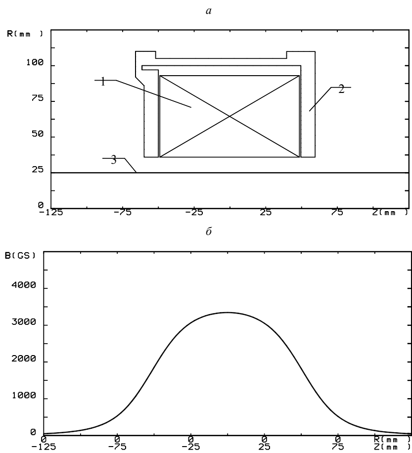
Рис. 9. Расчетная геометрия магнитной линзы (а) и осевое распределение магнитного поля B при максимальном токе в обмотке линзы 29,25 кА-витков (б). Цифрами обозначены: 1 – катушка с током, 2 – магнитный экран, 3 – контур трубки дрейфа.
