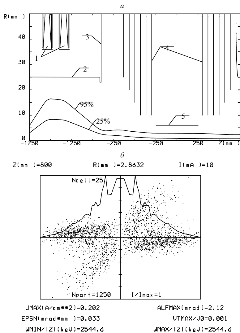
Рис. 11. Результаты расчета ионно-оптического тракта ускорителя-тандема для схемы «мягкой» фокусировки пучка H^- с током 10 мА и начальной энергией 25 кэВ: a – огибающие 25 % и 95 % тока пучка; b – радиальное распределение плотности тока и фазовый портрет пучка на выходе из ускорителя. Цифрами обозначены: 1 – магнитные линзы, 2 – трубка дрейфа, 3 – вакуумный бак, 4 – высоковольтный электрод, 5 – перезарядная трубка.
