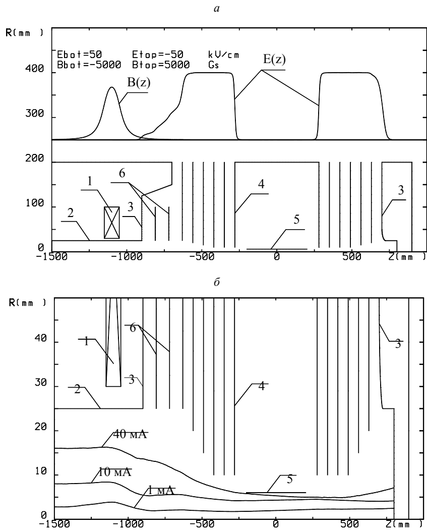
Рис. 6. Согласованный ввод 25 кэВ пучка H^- в ускоритель-тандем с использованием схемы «мягкой» фокусировки: геометрия ионно-оптического тракта, осевое распределение полей (а) и расчетные огибающие ионных пучков с током 1 мА, 10 мА и 40 мА, охватывающие 95 % тока (б). Цифрами обозначены: 1 – катушка с током, 2 – трубка дрейфа, 3 – вакуумный бак, 4 – высоковольтный электрод, 5 – перезарядная трубка, 6 – дополнительные электроды.
