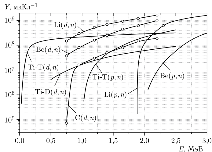
Рис. 1. Кривые полного выхода нейтронов основных нейтроногенерирующих ядерных реакций в зависимости от энергии на 1 мкКл налетающего пучка
