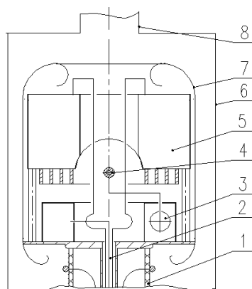
Рис. 7. Прототип ускорителя-тандема. 1 – проходной металлокерамический изолятор, 2 – стяжка-труба, 3 – газовый объем с натекателем, 4 – перезарядная трубка, 5 – азотная ловушка, 6 – "земляной" электрод, 7 – высоковольтный электрод, 8 – горловина насоса.
