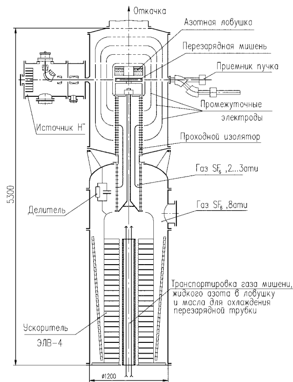
Рис. 1. Общий вид ускорителя-тандема.
