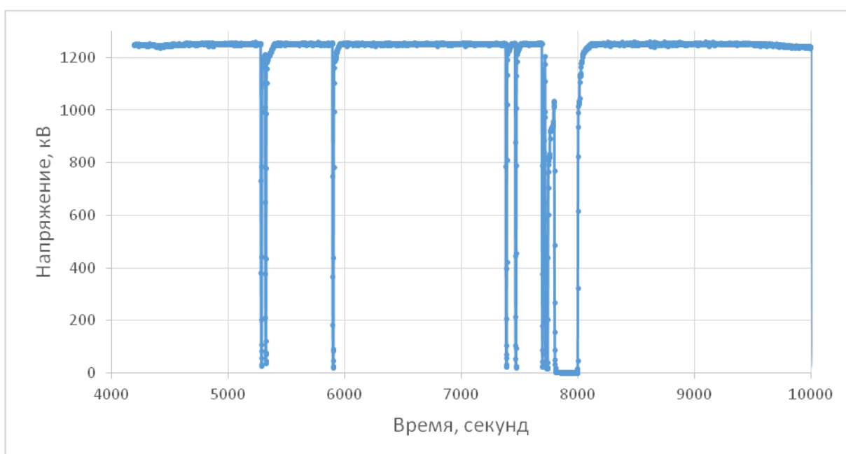
Рис. 21. Работа ускорителя при напряжении 1,25 МВ
