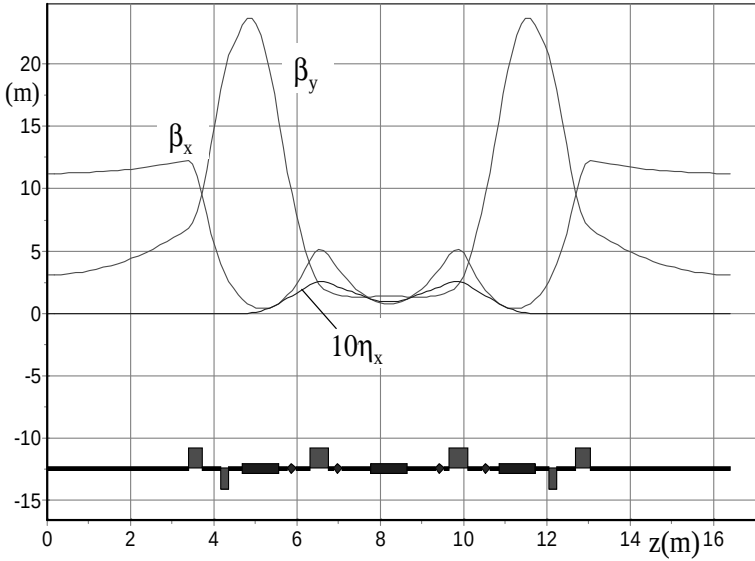
Fig. 5.10. Triple bend achromat [42]
