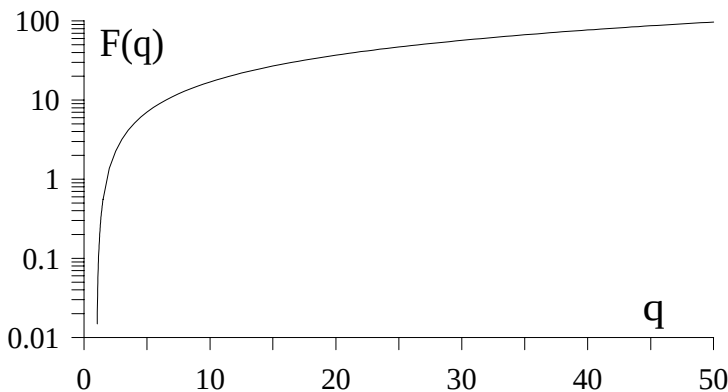
Fig. 6.12. Over voltage function F(q)
